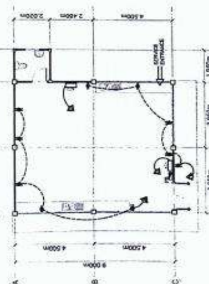
2 POWER LAY-OUT SCALE: 1/32
